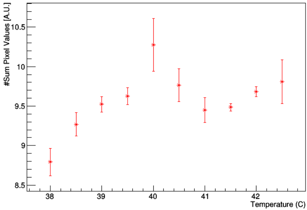
CMOS- thermal noise
